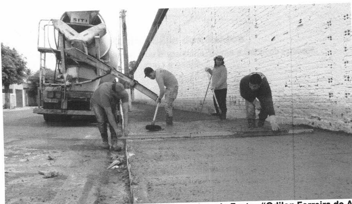
FOTO 26 – Concretagem de passeio público no Recinto de Festas "Odilon Ferreira de Almeida"
